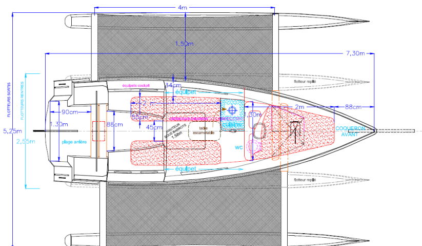
ASTUS 24 - aménagements
